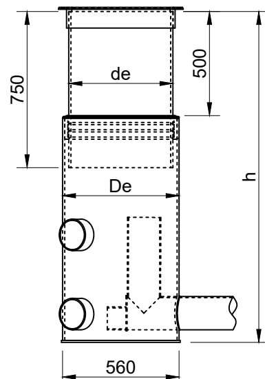
VIRTAUKSENSÄÄTÖKAIVO
