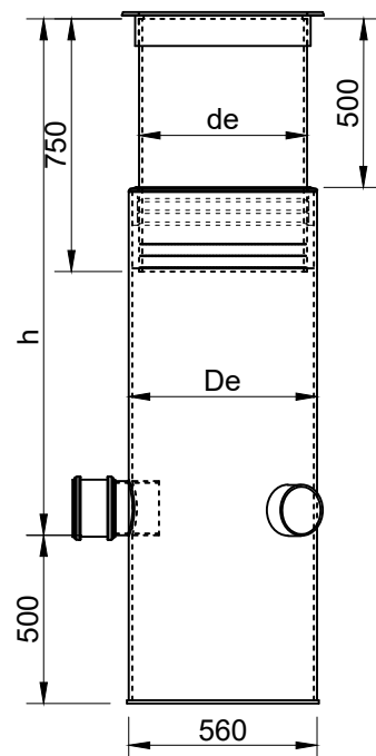
HIEKANEROTUSKAIVO
